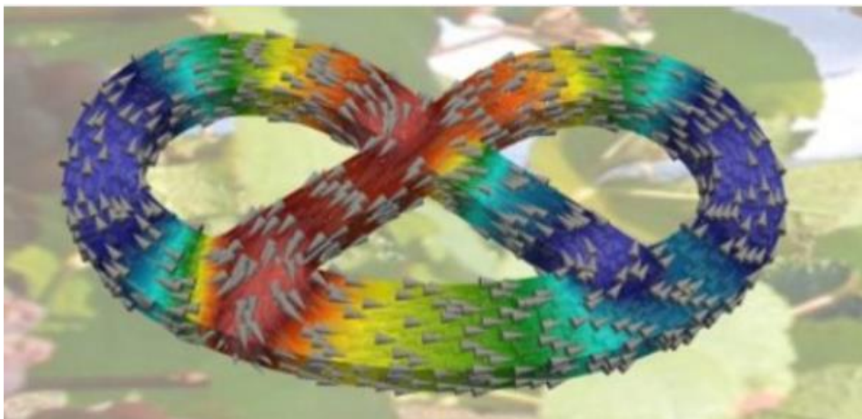
FIGURE 1. Bretzel micromagnétique (sur fond de vignoble) copyright R. Hertel
